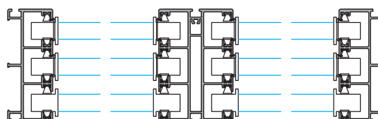
Sección Vertical
