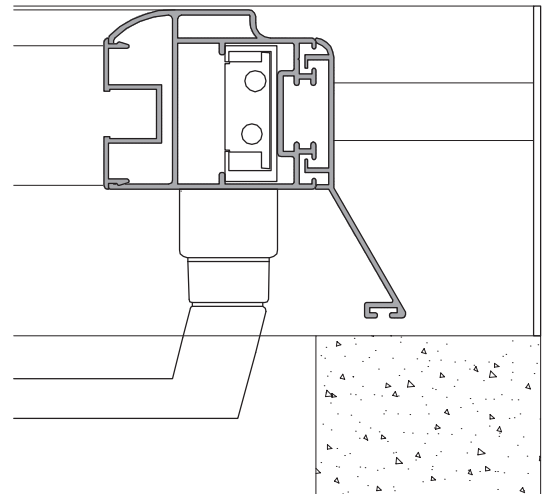
Sección Horizontal
