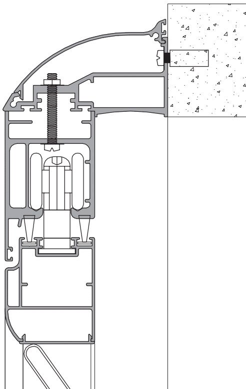
Sección Vertical
