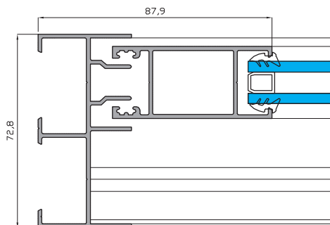
Sección Horizontal
