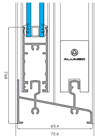
Sección Vertical
