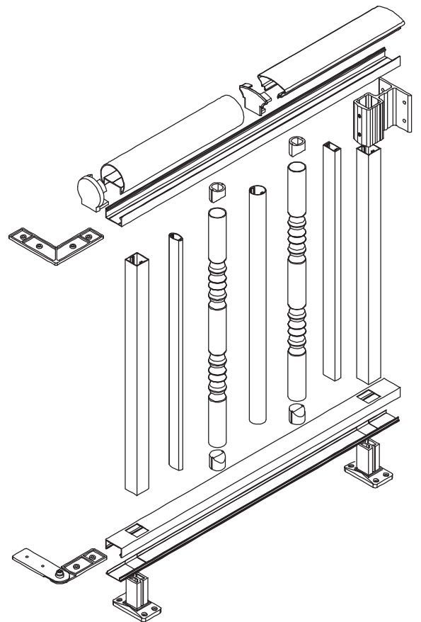
BARANDILLA CONVENCIONAL
